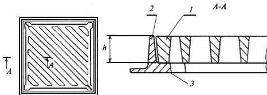
Рисунок Б.1 - Дождеприемник ливнесточного колодца
